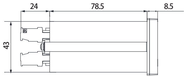
侧视图
