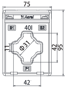
正视图
