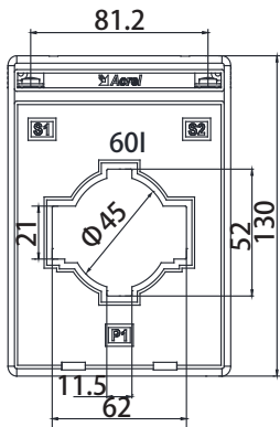
正视图
