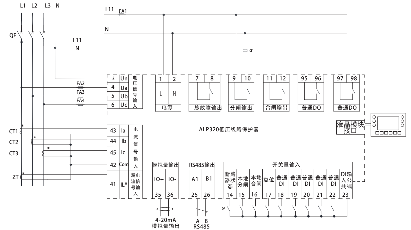
ALP320低压线路保护器应用方案图
