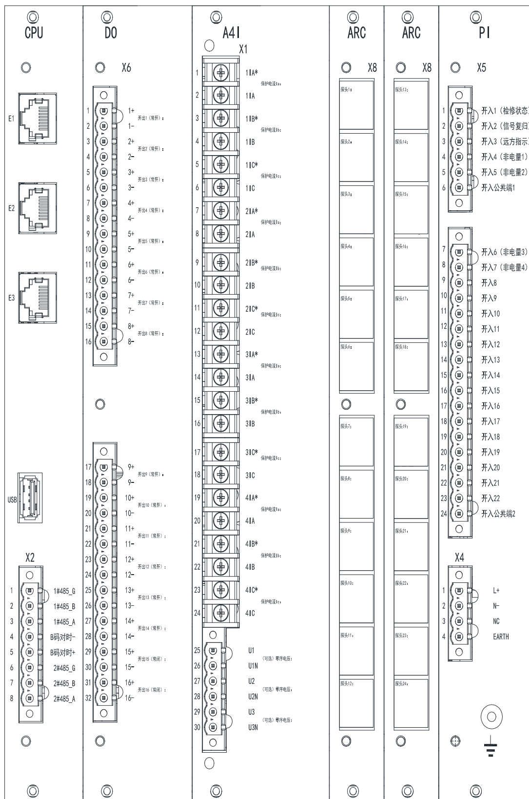
图 3.2 ARB6-A24 背板端子定义图
