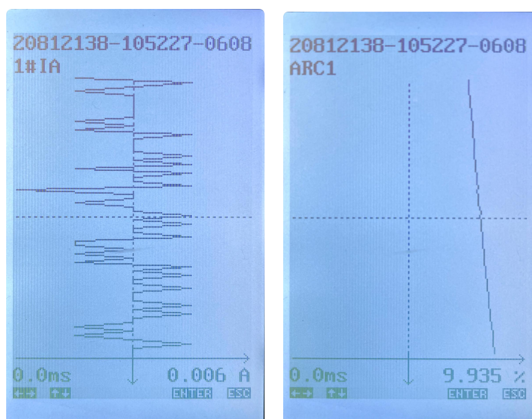
图 4.27 录波数据
