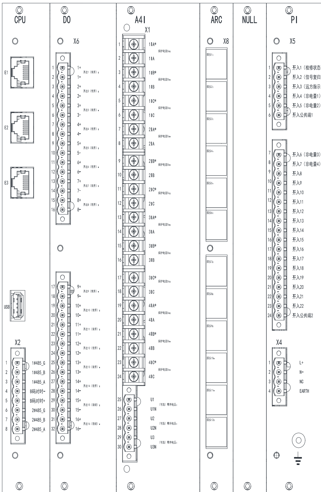
图 3.4 ARB6-A12 背板端子定义图
