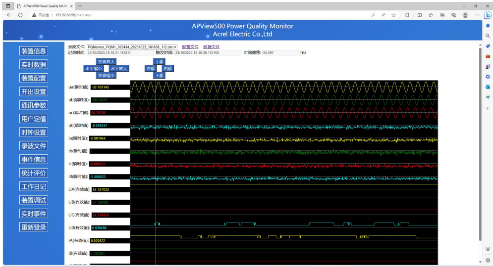
图 1.4 波形界面
