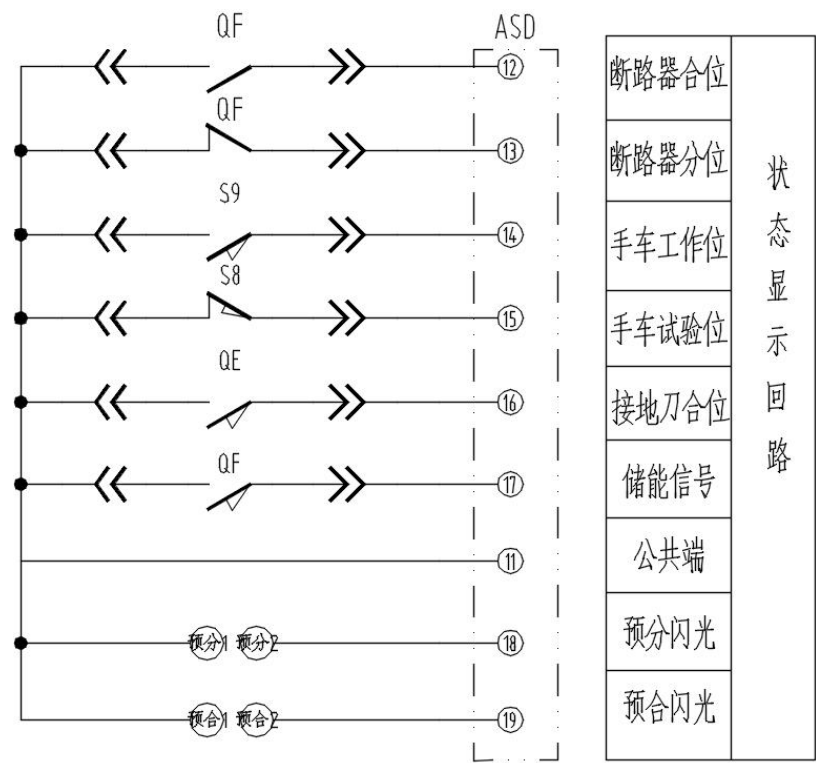
图 1.11 ASD 开关量输入回路典型接线图
