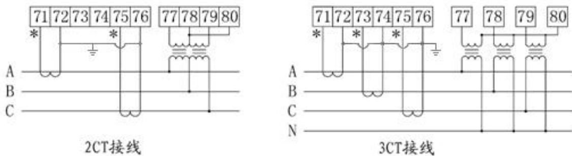
图 2.4 接线方式
