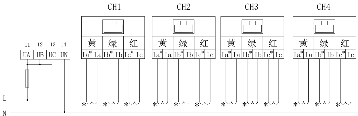
图 9 单相电压、电流直接接入
