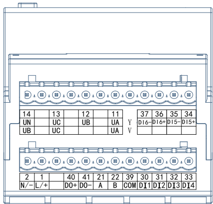
图6 DTSD1352-4S (6DI1DO) 模块反面接线端子
