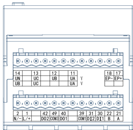
图4 DTSD1352-4S (2DI2DO) 模块反面接线端子
