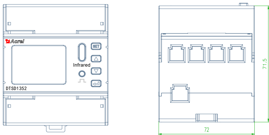
图2 DTSD1352 - 4S 尺寸图 表4 DTSD1352 - 4S 模块尺寸
