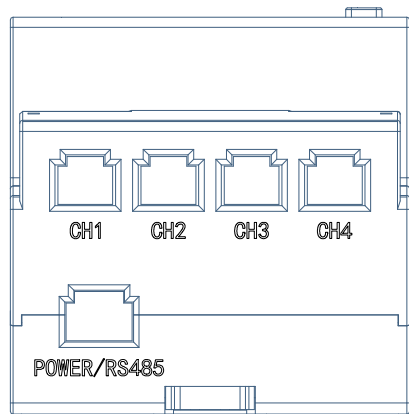
图5 DTSD1352-4S (6DI1DO) 模块正面接线端子
