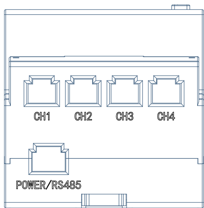
图3 DTSD1352-4S (2DI2DO) 模块正面接线端子
