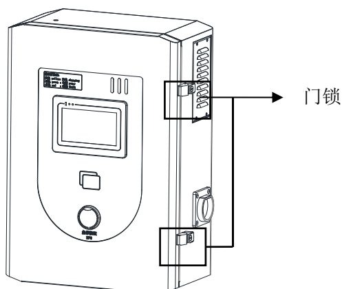
图 3-12 门锁位置
