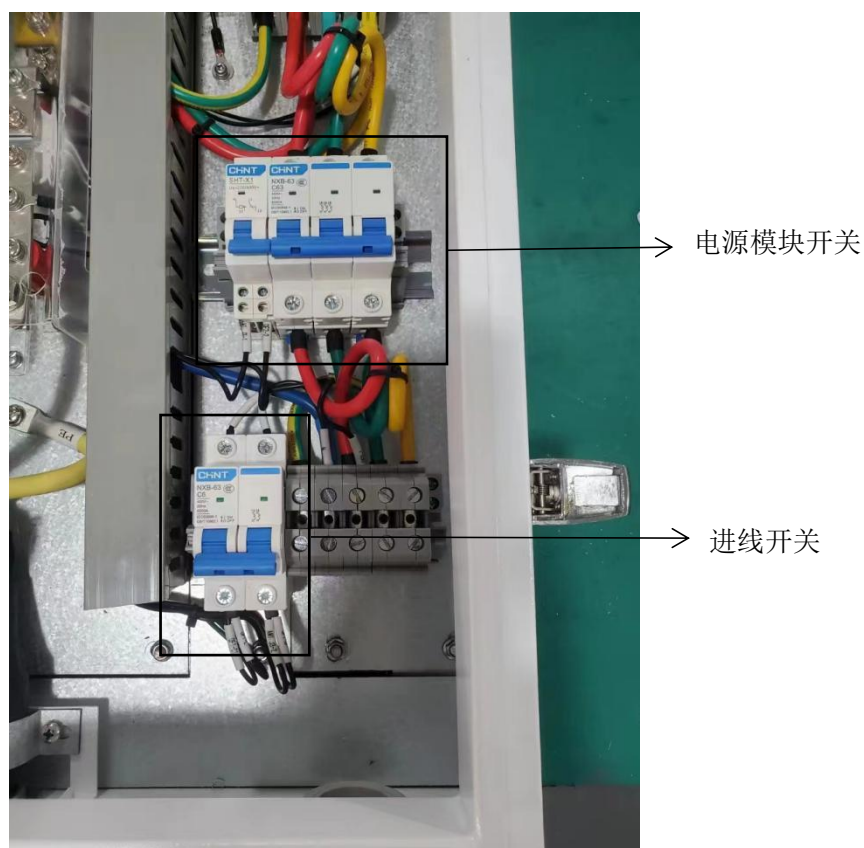
图 5-1 开关位置
