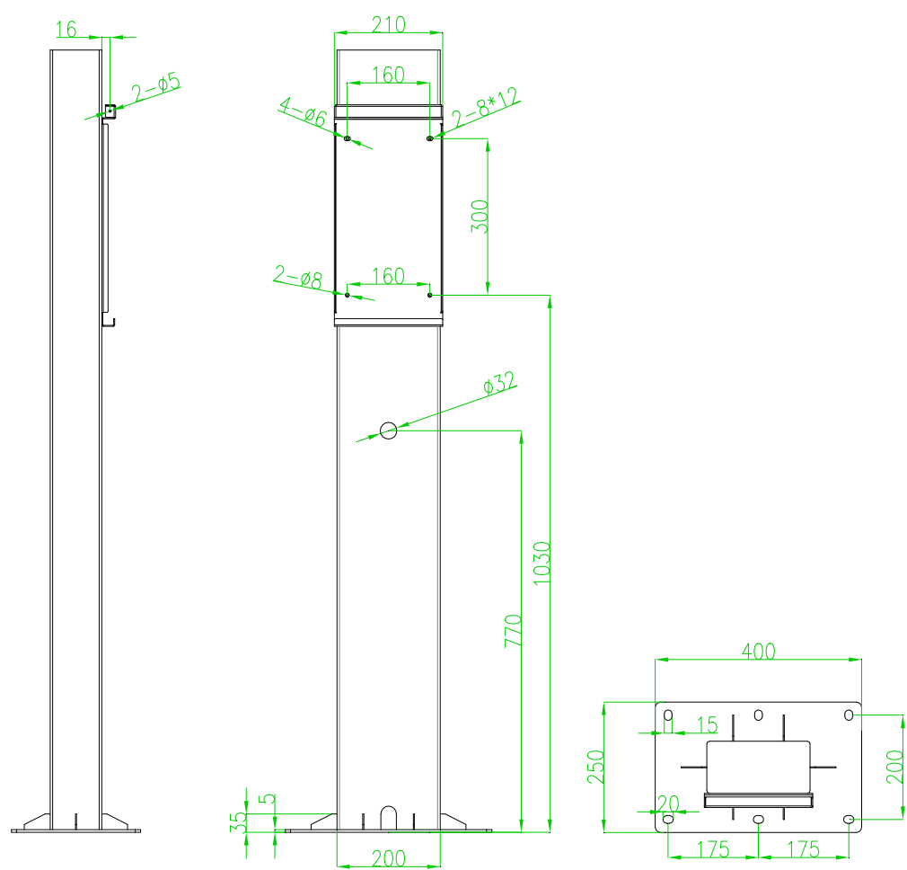
图 3-8 立柱尺寸
