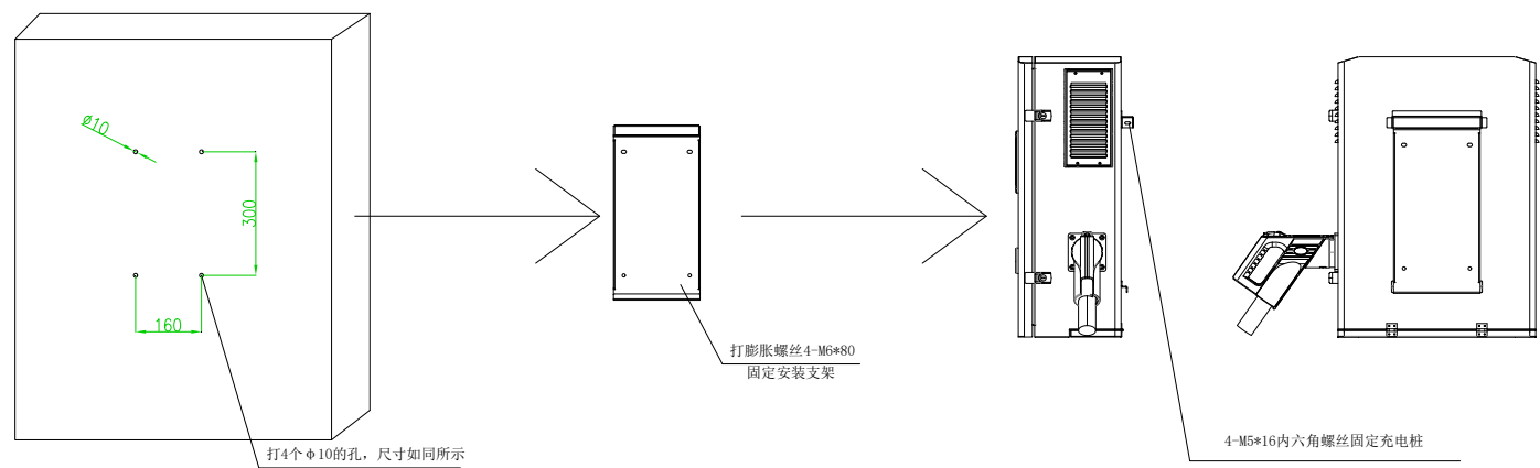
图 3-7 壁挂充电机安装顺序
