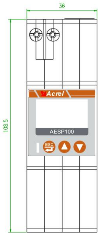
图2 智能网关外形尺寸图
