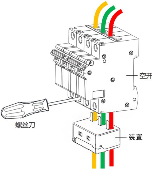
图5 装置接线示意图
