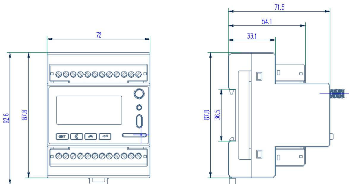
图 2 ADW300 尺寸图
