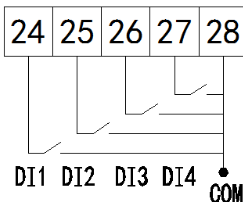
开关量输入
