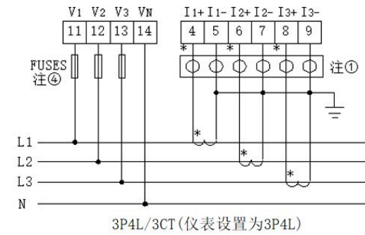
3P4L/3CT (仪表设置为3P4L)
