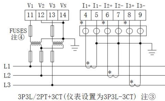
3P3L/2PT+3CT (仪表设置为3P3L-3CT) 注③
