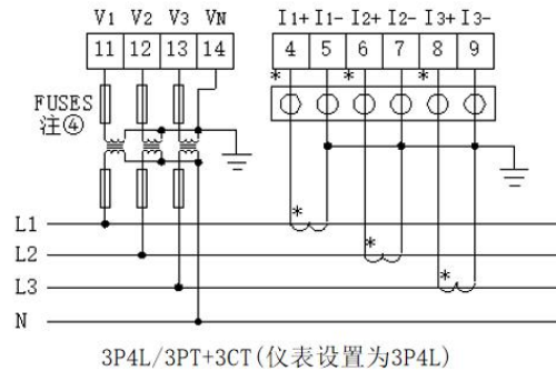
3P4L/3PT+3CT (仪表设置为3P4L)
