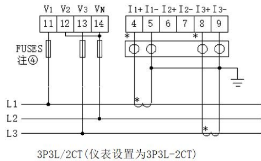
3P3L/2CT (仪表设置为3P3L-2CT)
