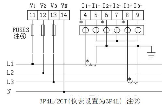
3P4L/2CT (仪表设置为3P4L) 注②
